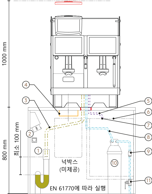
빈 호퍼를 보충/제거하는 데 필요한 최소 높이
